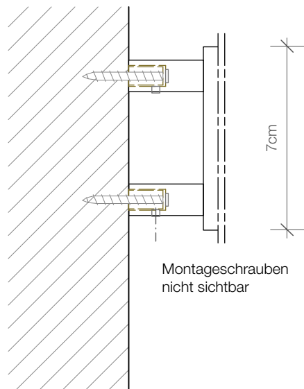
Schnitt Section
